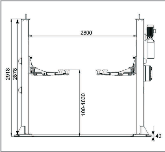
Boyut Ölçüleri Çizimi
