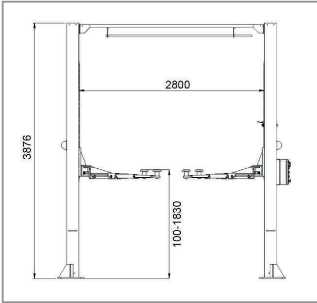
Boyut Ölçüleri Çizimi
